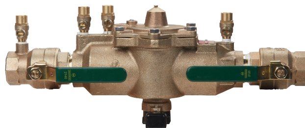
LF009-FS
